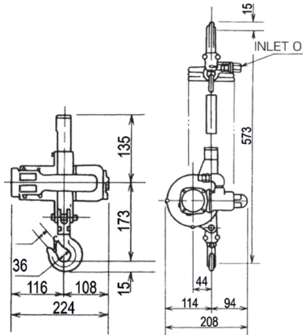
TMM-140AE
